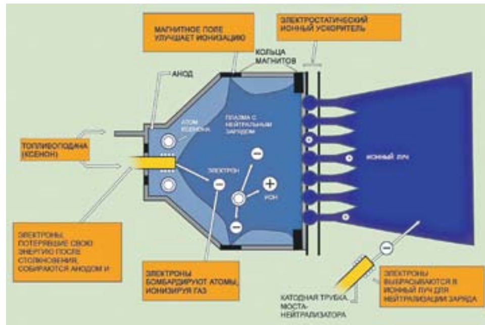
Схема ионного двигателя с сайта lab-37.com
